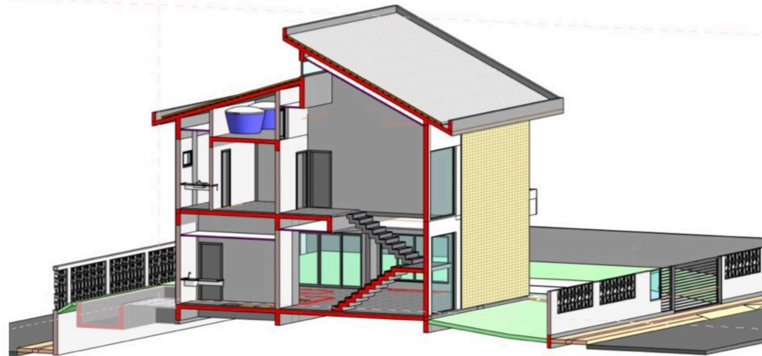
BIM System . LOD 400 | RESIDÊNCIA FHS
